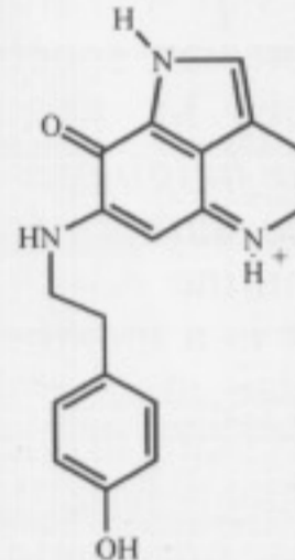
32 Makaluvamine D
