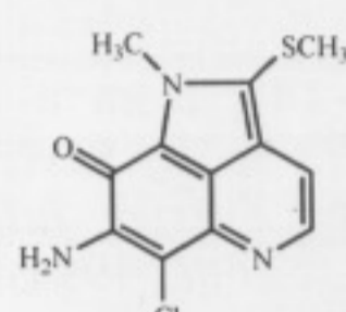
26 Isobatzelline D
