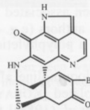
42 Prianosin B
