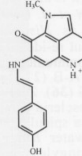
33 Makaluvamine E
