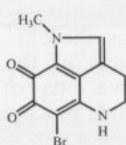
35 Makaluvone
