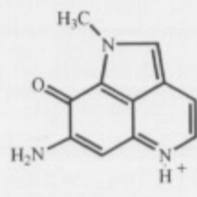
31 Makaluvamine B
