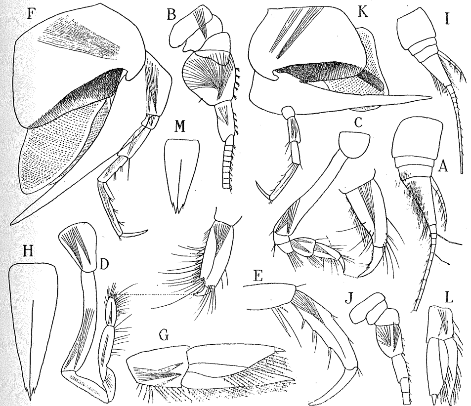
FIG. 2. — Cyphocaris Alicei nov. sp. Mâle : A, antenne supérieure; B, antenne inférieure; C, gnathopode antérieur; D, gnathopode postérieur; E, derniers articles d'une patte de la troisième paire; F, patte de la cinquième paire; G, uropode de la dernière paire; H, telson. — Femelle : I, antenne supérieure; J, antenne inférieure; K, patte de la cinquième paire; L, uropode de la dernière paire; M, telson. (Toutes les figures sont dessinées avec le même grossissement).
