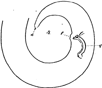
4 Hinterende des Männchens von Enoplus cirrhatus .
