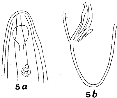
Fig. 5. Leptosomatum bacillatum (EBERTH) a. Anterior end, b. Tail, \times 225
