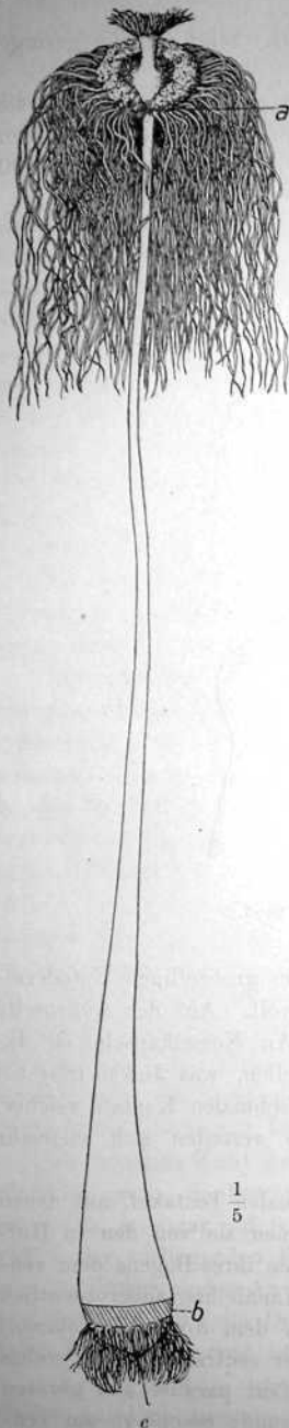
Fig. 2. Gesamtansicht mit Zuwachszonen, a der Mund-scheibe; b der Wurzelhaare; c des gesamten Hydrocaulus.
