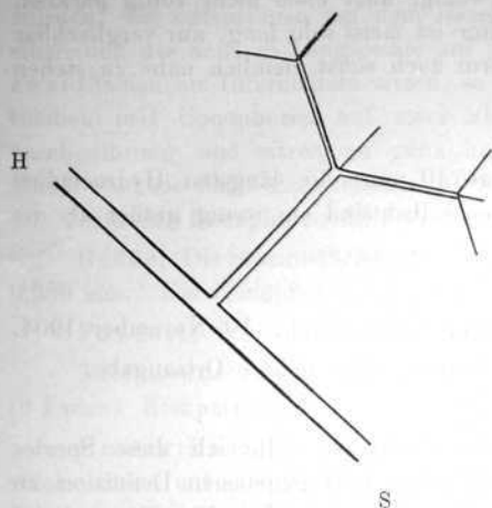
Fig. 8. Halicornaria expansa Jäderholm. Schema der Verzweigung. HS = Hauptstamm. Die Hydrocladien sind weggelassen.
