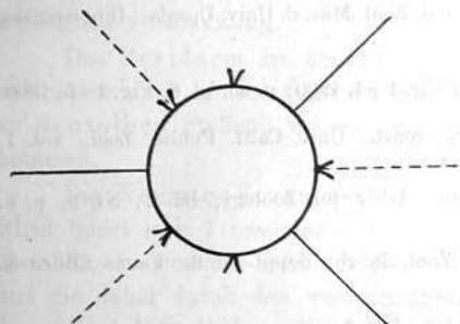
Fig. 5. Antennularia japonica n. sp.
