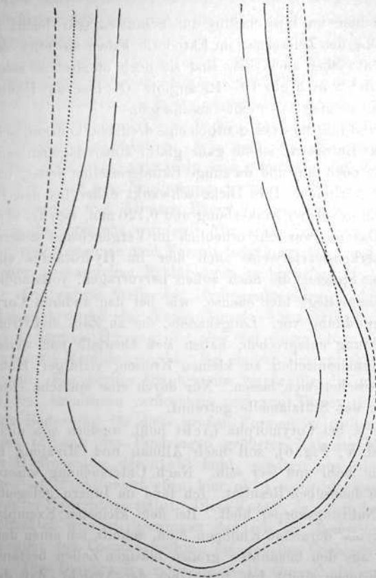
Fig. 4. Profile der Wurzelknollen. (Natürliche Größe.)
