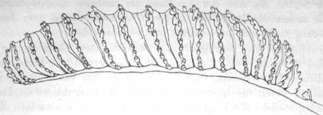
Fig. 6. Aglaophenia Suensonii Jäderholm. Corbula. Vergr. 20:1.
