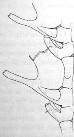
Fig. 7. Aglaophenia laxa Allman. Varietät mit langen Nematophoren. Vergr. 75:1.
