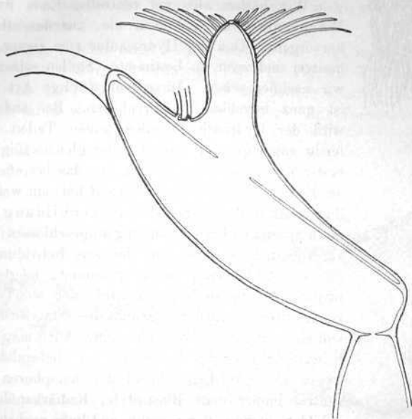
Fig. 1. Medianchnitt, nat. Größe (nach Miyajima mod.).
