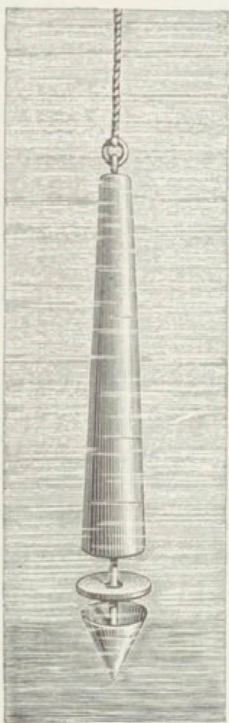
Fig. 3. — Plomb de sonde à coupe.
