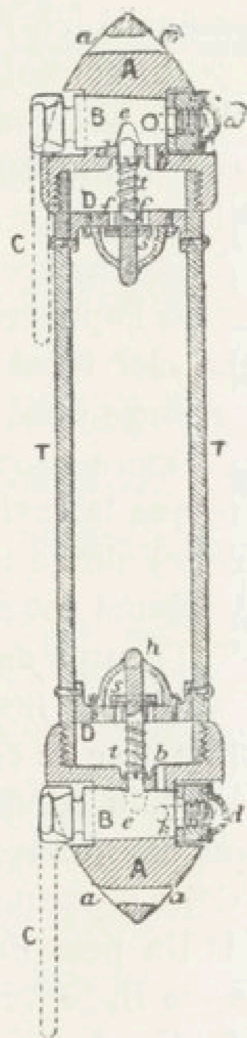
Fig. 21. — Bouteille à eau.
