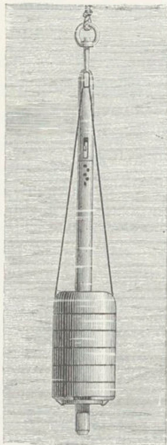
Fig. 7. — Sondeur du Challenger .
