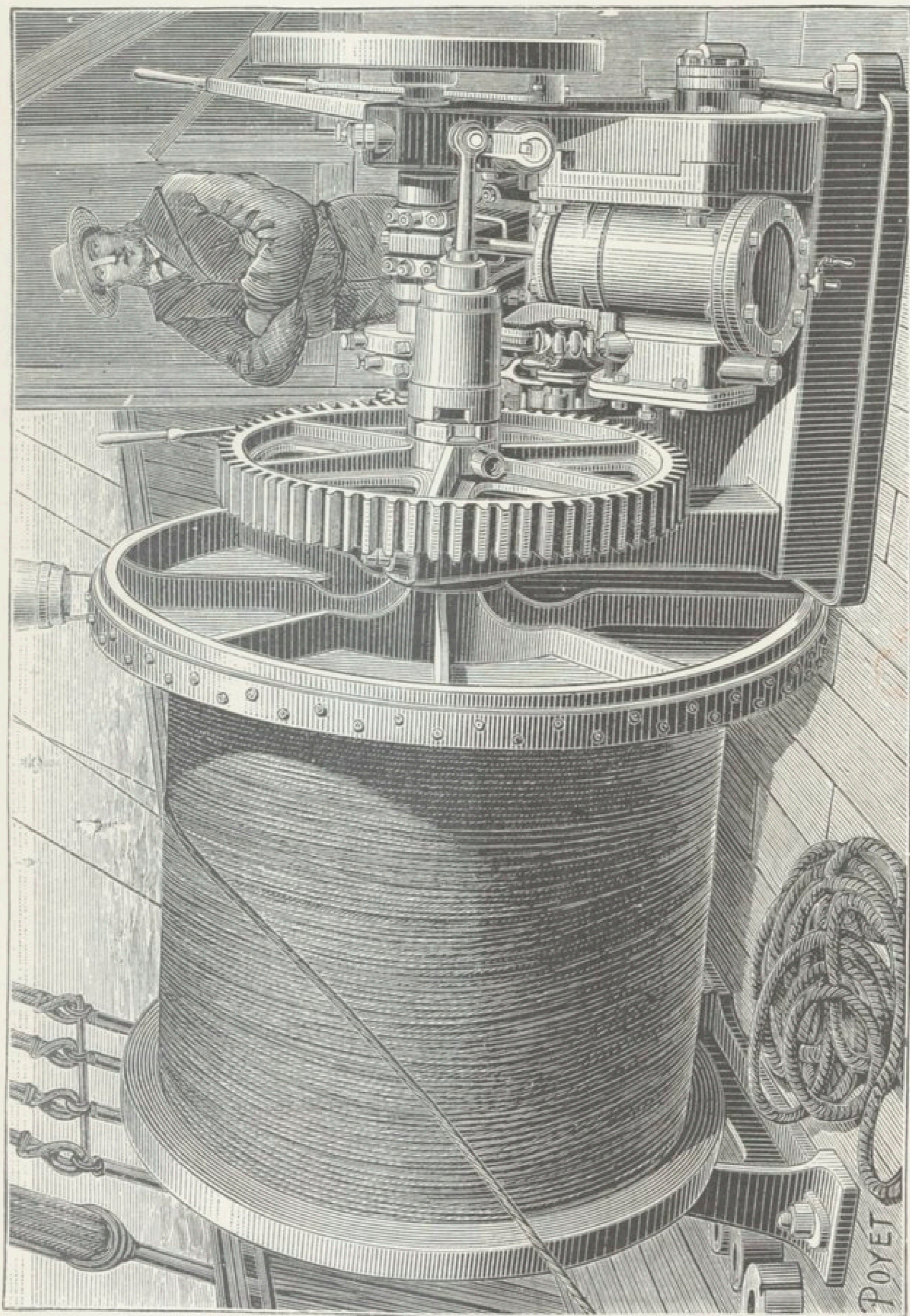
Fig. 17. — Treuil pour enrouler le câble d'acier (d'après une photographie).
