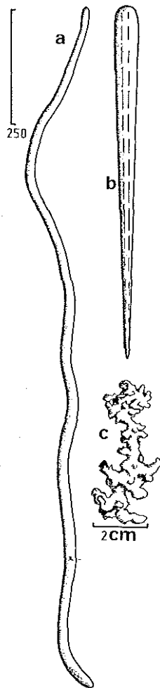
FIGURE 53. Acanthella vaceleti n. sp., a. sinuous strongyle, b. style, c. habit.
