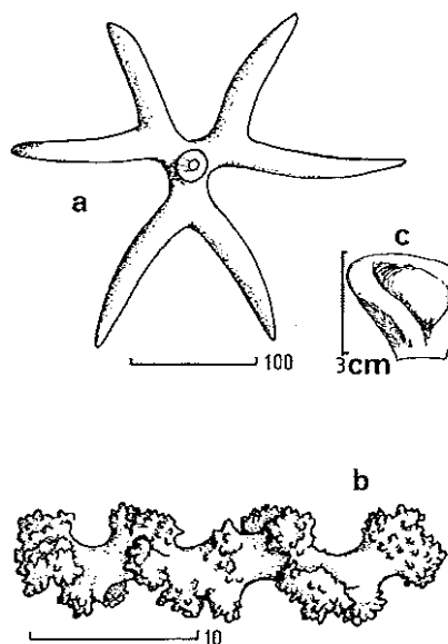
FIGURE 25. Corallistes paratypus n. sp., a. ectosomal dichotriaene, b. spiraster, c. habit.
