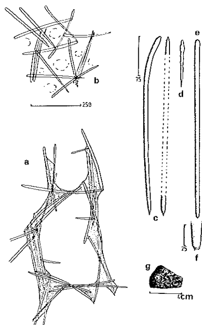
FIGURE 60. Echinochalina melana n. sp., a. choanosomal skeleton, b. tangential view of ectosome, c. stylote megascleres, d. echinating acanthostyle, e. inequidended strongylote megasclere, f. acanthose apex of strongylote, g. habit.
