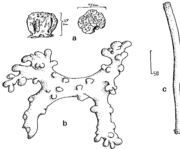
FIGURE 29. Aciculites higginsi , a. habit, b. desma, c. ectosomal anisostrongyle.
