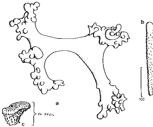
FIGURE 30. Aciculites cribrifera , a. desma, b. ectosomal acanstrongyle, c. habit.
