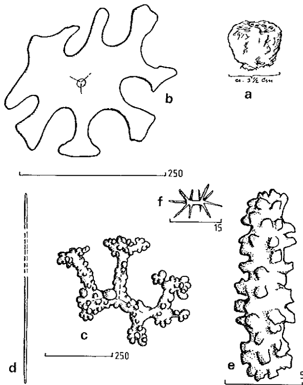
FIGURE 23. Racodiscula asteroides , a. habit, b. ectosomal discotriaene, c. desma, d. oxeote, e. acanthorhabd, f. amphiaster.
