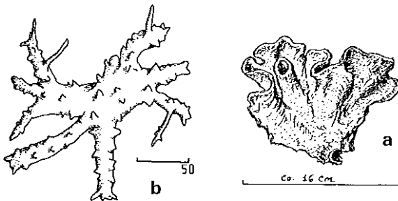
FIGURE 34. Vetulina stalactites , a. habit, b. desma.
