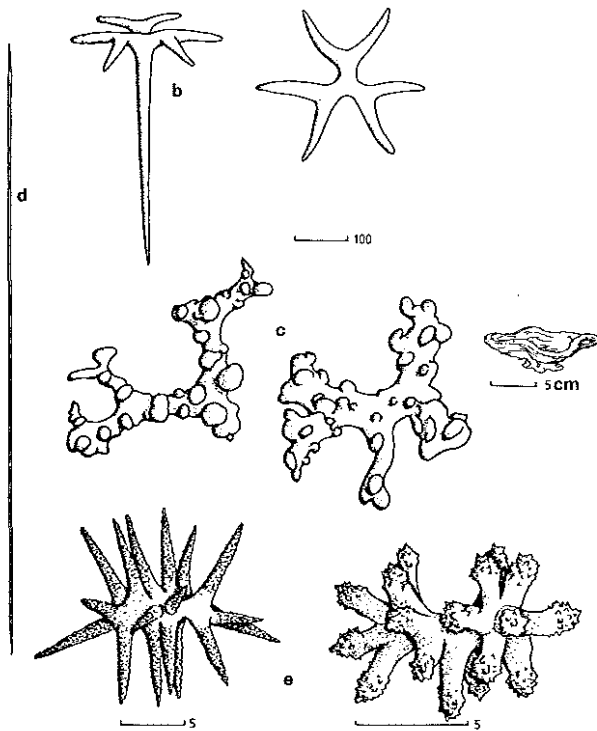
FIGURE 24. Corallistes typus , a. habit, b. ectosomal dichotriaenes, c. desmata, d. oxecote, e. spiraster/amphiaster.
