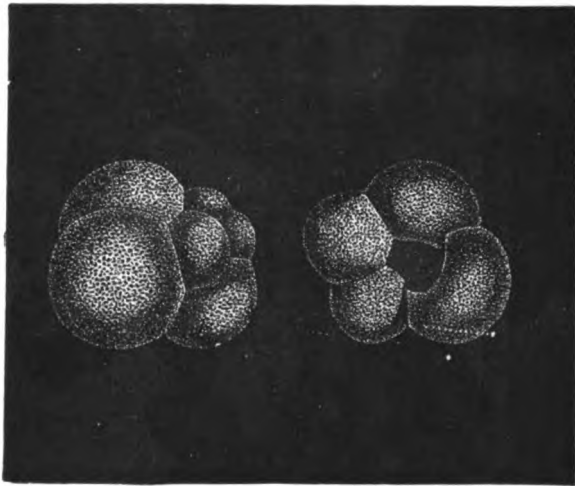
Fig. 156. — Globigérines.
