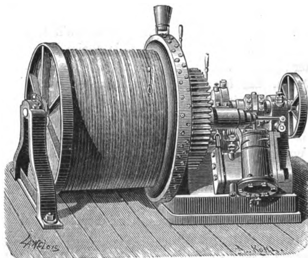
Fig. 51. — Treuil servant à enrouler le câble d'acier.
