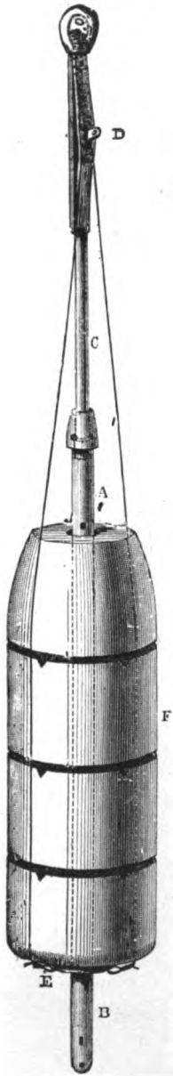
Fig. 44. — L'Hydre , sondeur du Porcupine , employé aussi au début de la campagne du Challenger .
