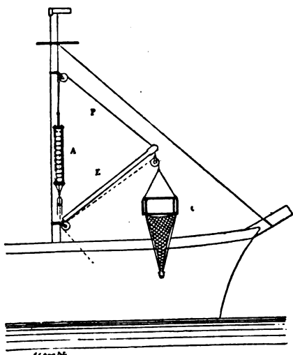
Fig. 56. — L'accumulateur supportant la poulie du chalut à bord du Talisman .
