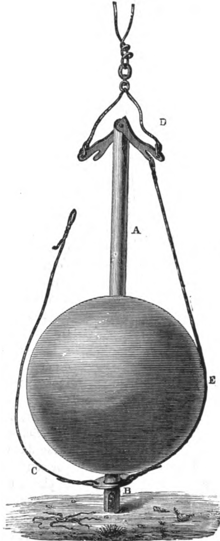
Fig. 41. — Sondeur de Brooke arrive au fond, au moment où le poids se détache.
