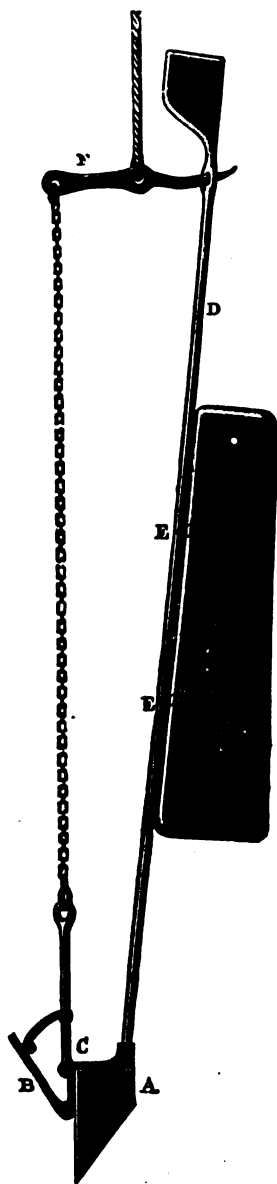
Fig. 42. — Sondeur du Lightning .
