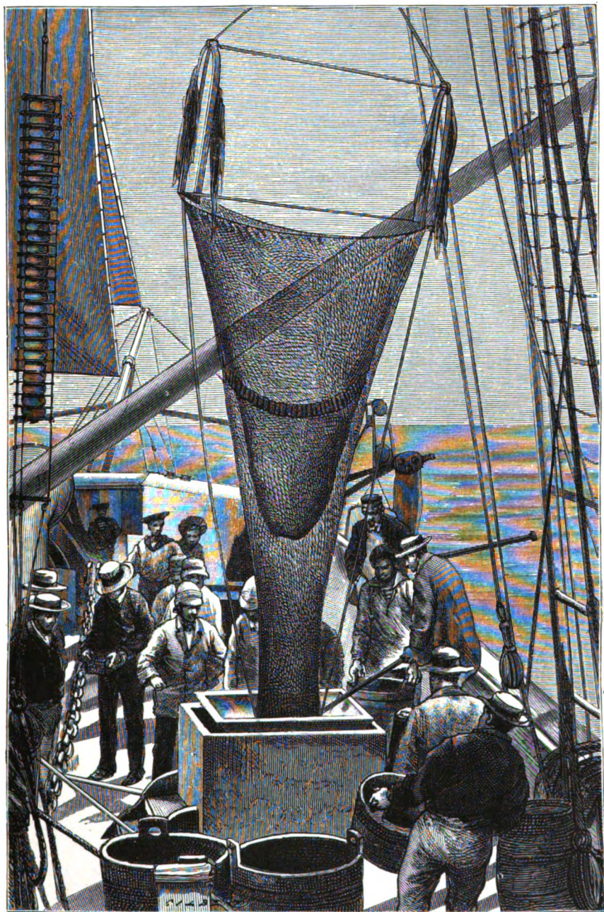
Fig. 53. — Retour du chalut à bord du Talisman . (D'après une photographie de M. le professeur Léon Vaillant.)
