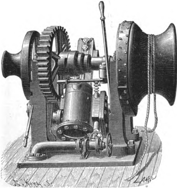
Fig. 55 — Treuil employé pour remonter la drague.
