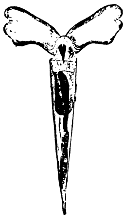
Fig. 128. — Cuvieric.
