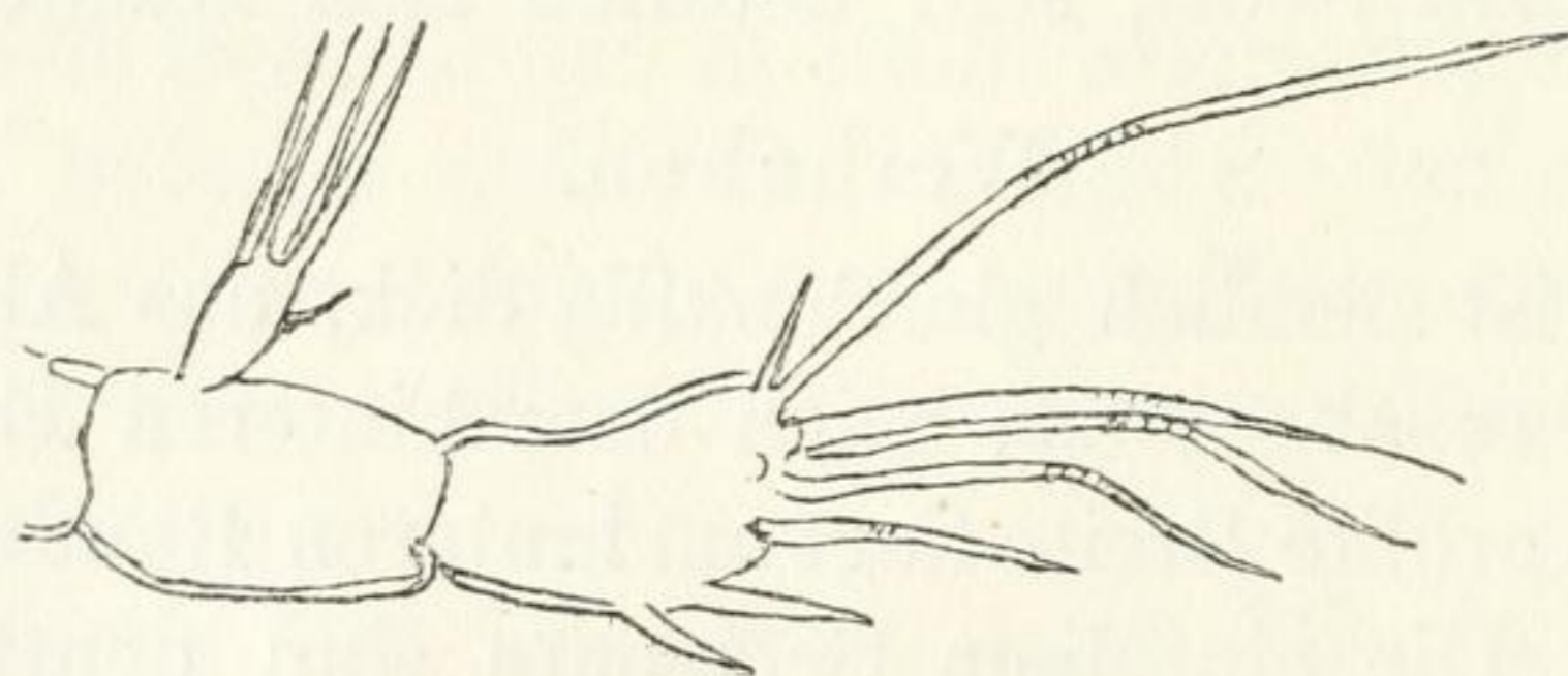
Fig. 1. Furca ♀, dorsal.
