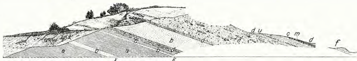
Fig. 2. a Ton, b feinkörniger Sand, d sandiger Ton, e grobkörniger, kleinschotteriger Sand mit Sandsteinkonglomerationen, f Rhyolittuff, x untere fossilarme Sandschicht, k fossilreiche Sandschicht, u sandiger Ton mit Unio sp. und Cyrenen-Steinkörnern, c Cerithienschicht, m Mytilenschicht.
