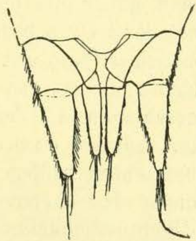
Fig. D. Trichoniscoides albidus var. topiaria GRAEVE. ♀. (No. 139 Rheinbreitbach.) Pleotelson mit den Uropoden. 78:1.
