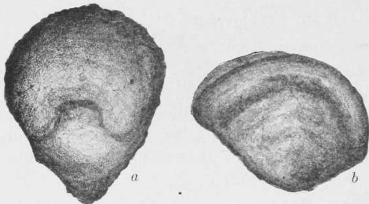
FIG. 20.—TEXTULARIA ABBREVIATA. \times 60 . a, APERTURAL VIEW; b, FRONT VIEW.
