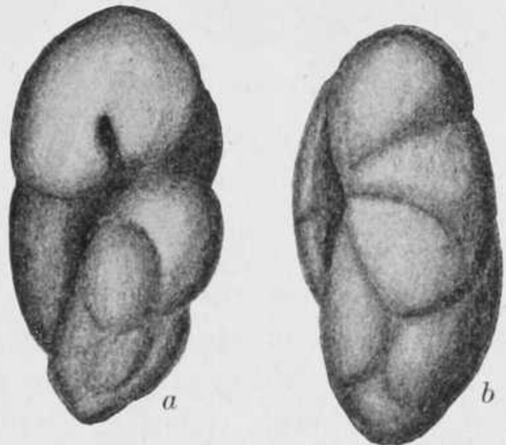
FIG. 142. BULIMINELLA SUBTERES. \times 80 . a, APERTURAL VIEW; b, SIDE VIEW.
