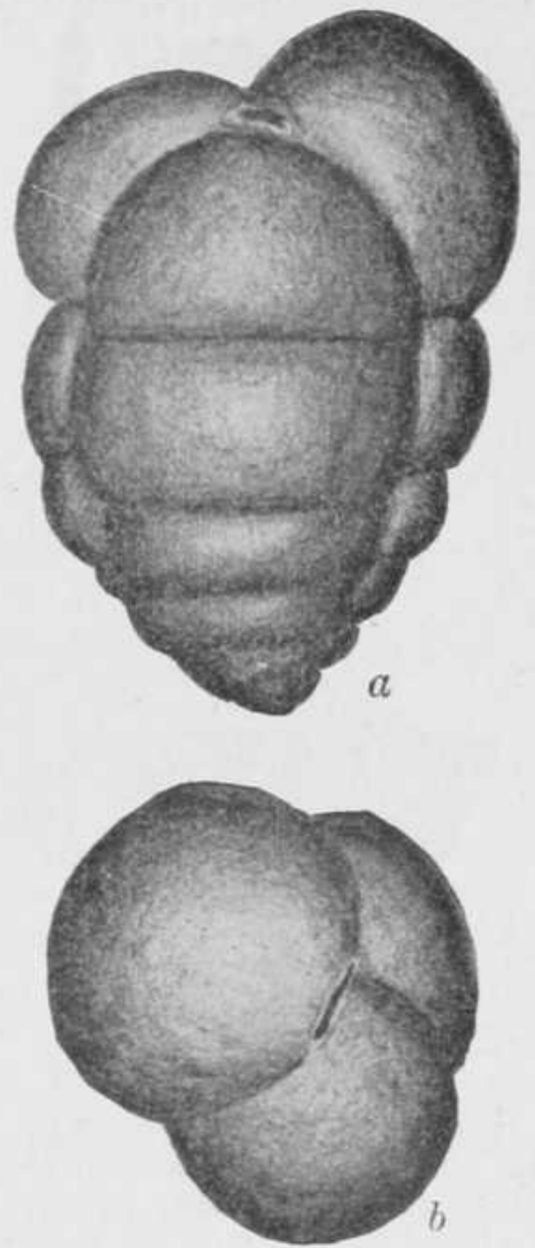
FIG. 87.—VERNEUILINA BRADYI. × 40. a, FRONT VIEW; b, APERTURAL VIEW.
