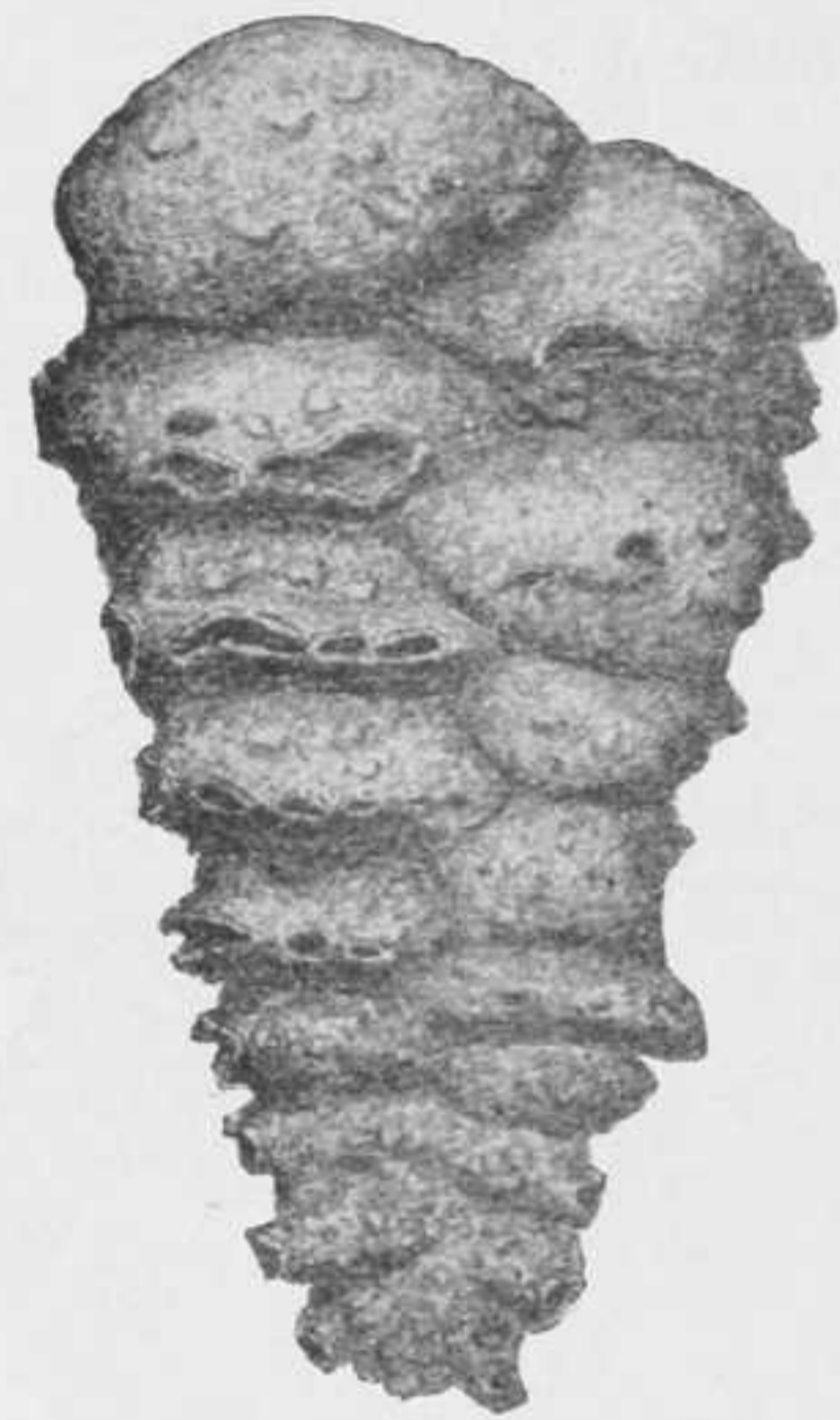
FIG. 11.—TEXTULARIA AGGLUTINANS, VAR. FISTULA. \times 40 .
