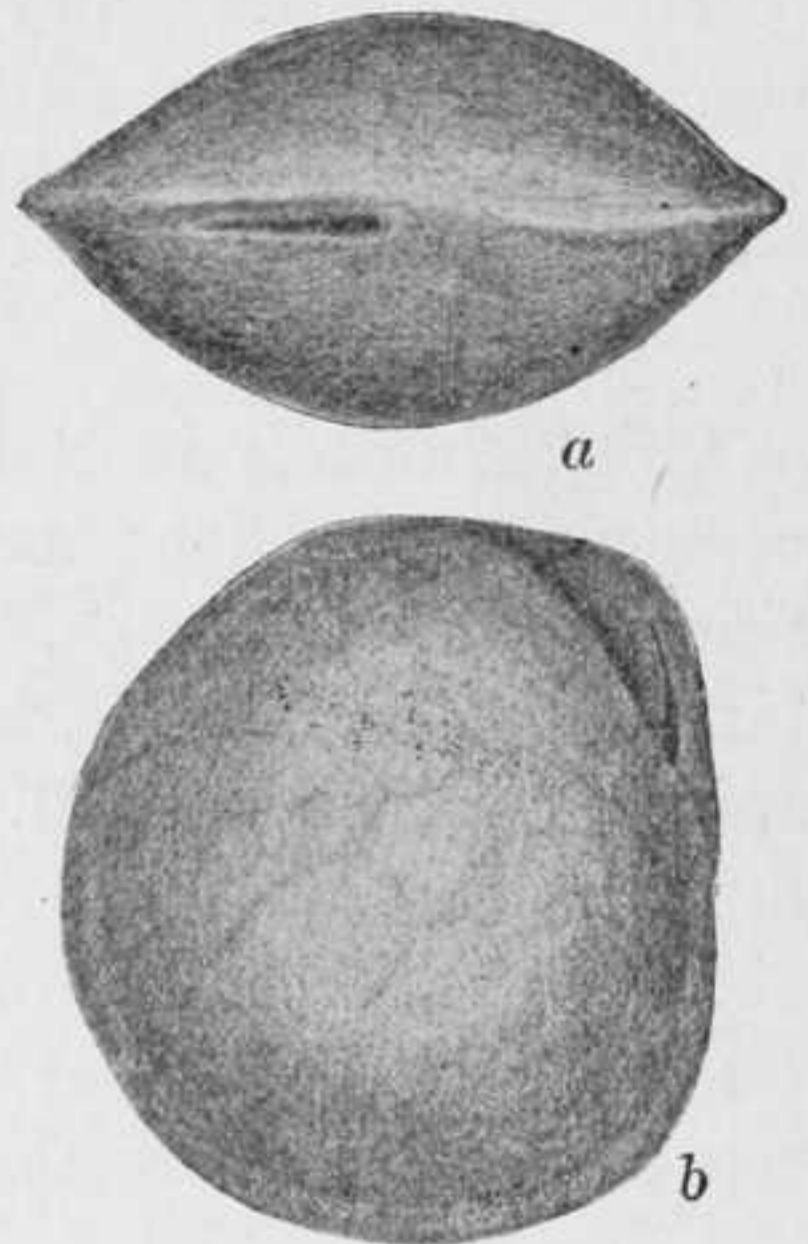
FIG. 150.—CASSIDULINA LÆVIGATA. X 30. a , APERTURAL VIEW; b , FRONT VIEW.
