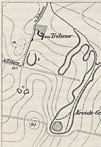
Kalkgruben bei Tribsov.
