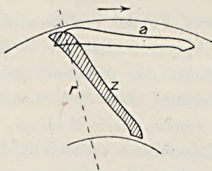
Längsschnitt durch die Wohnkammer eines Aspidoceras longispinum , ein Stück seitlich von der Sagittalebene.
